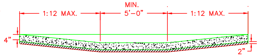
MIN 2" D.G.A. SECTION A-A
