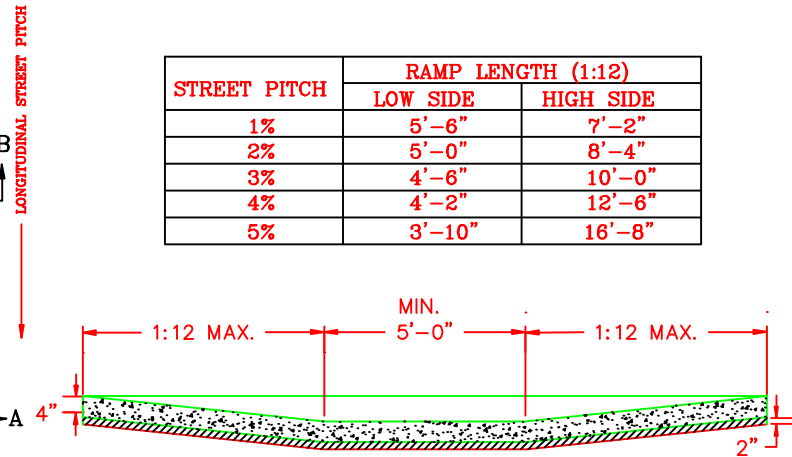
MIN 2" D.G.A. SECTION A-A
