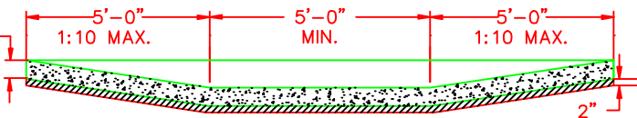
MIN 2" D.G.A. SECTION A-A
