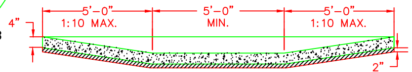
MIN 2" D.G.A. SECTION A-A
